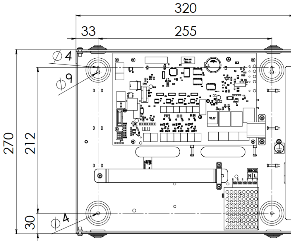
Рис.2. Габаритные и установочные размеры АПКП и ВПУ.
