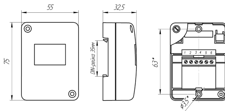
Рис.1. Габаритные и установочные размеры МШ-1.
