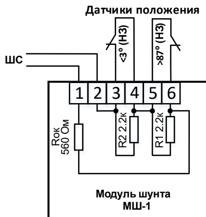
Рис. 2. Схема подключения модуля к контрольному шлейфу МАКС-У, МАКС-УРП.
