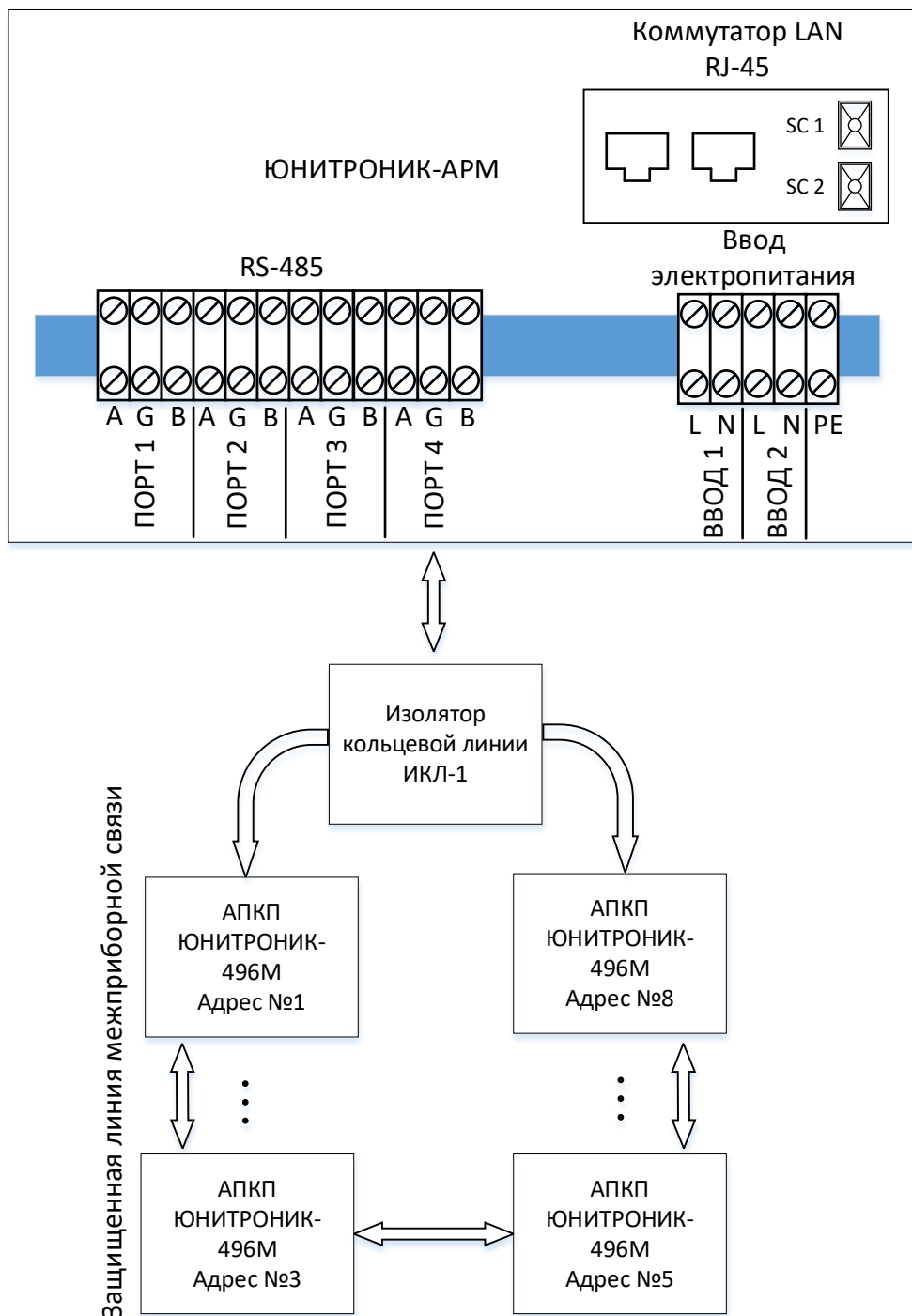
Рис.2. Расположение клемм и подключения АПКП «Юнитроник 496М» к АРМ. Изолятор кольцевой линии ИКЛ-1 рекомендуется размещать внутри корпуса АРМ.
