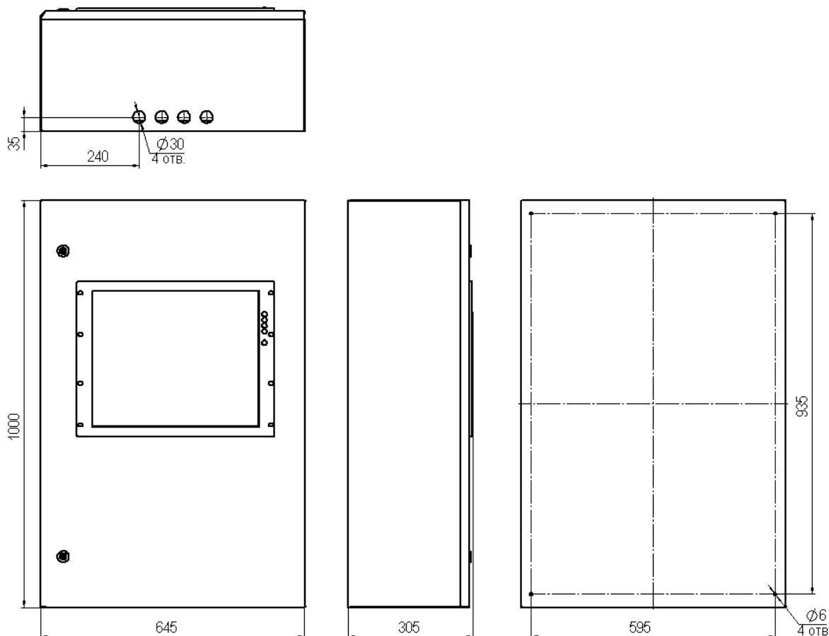
Рис.1. Габаритные и установочные размеры АРМ.
